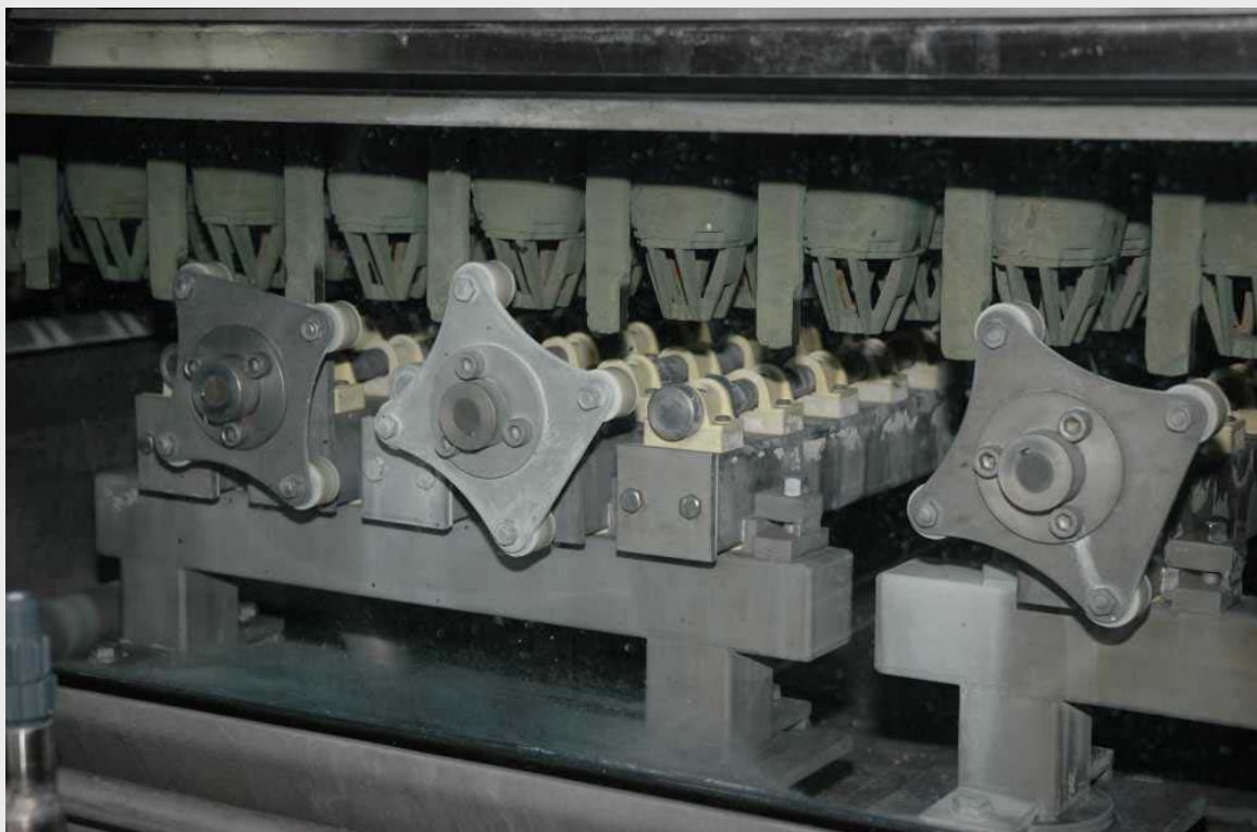
Бутылкомоечная машина – детальное фото
